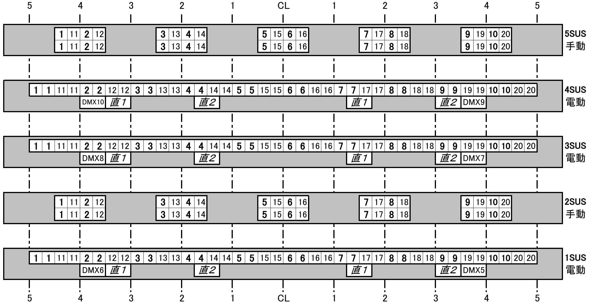
防府市公会堂 照明用サスペンションライト回路配置図(C20Aコン×2口 = DIM:3KW)
