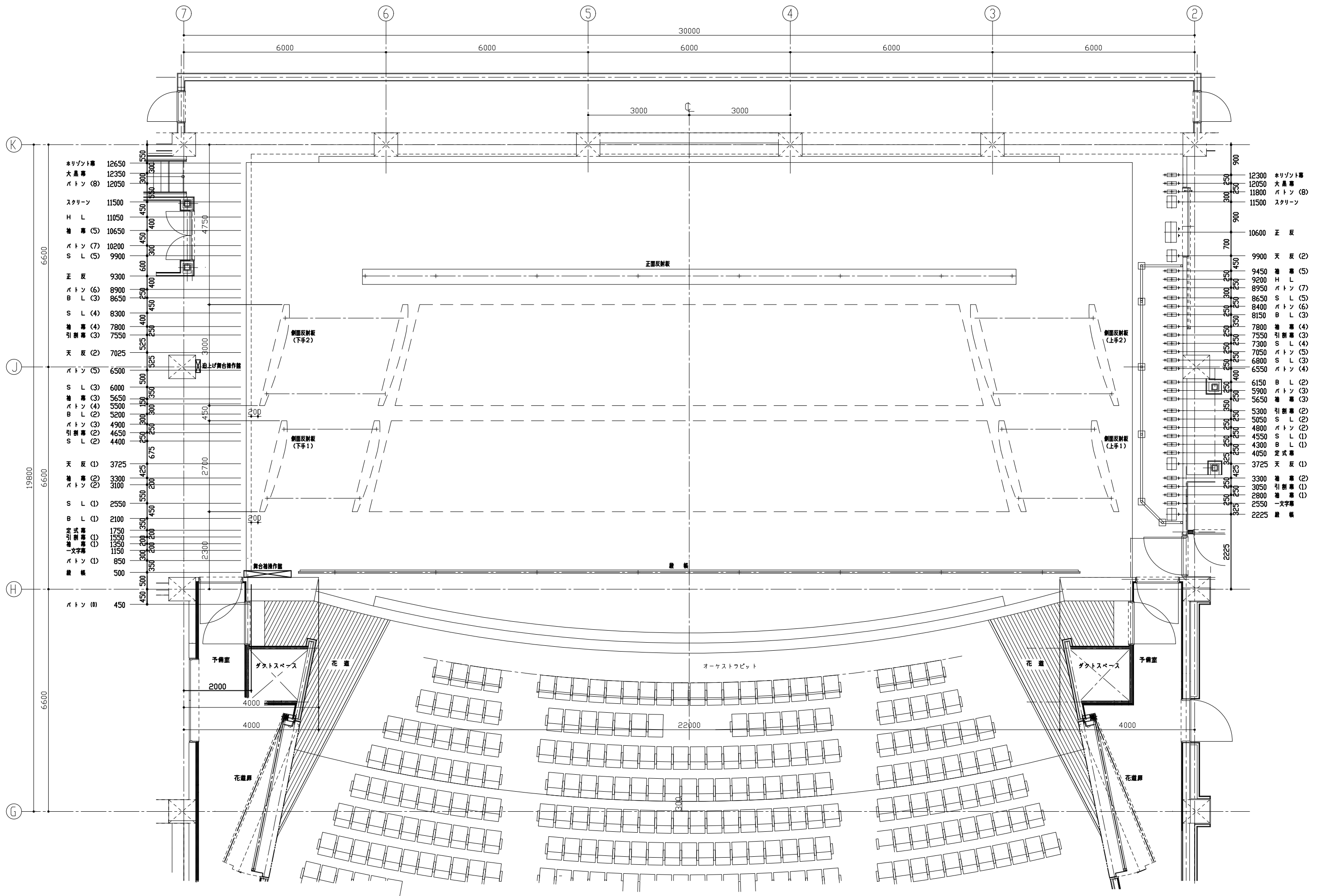
平面図 S=1:50
