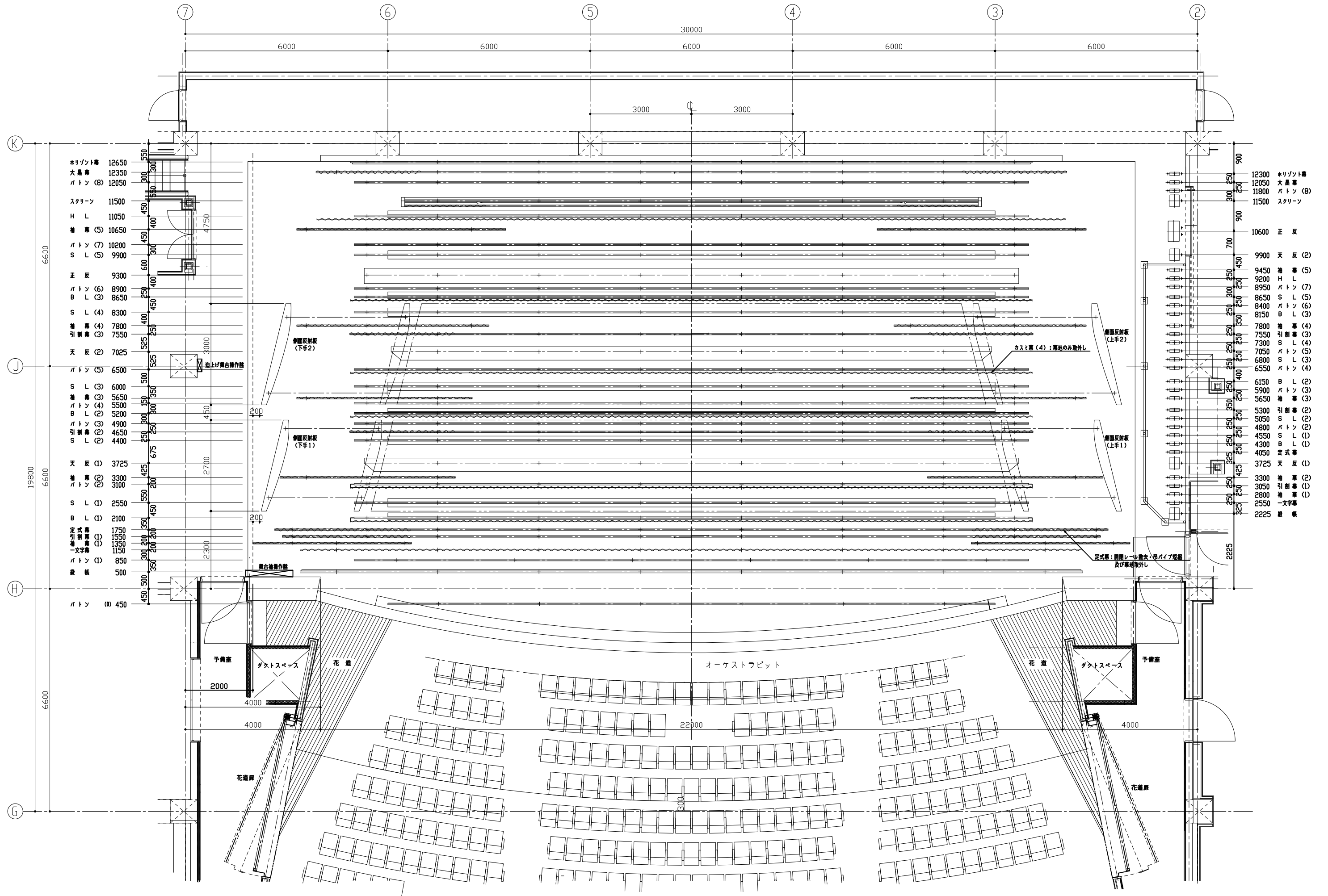
平面図 S=1:50
