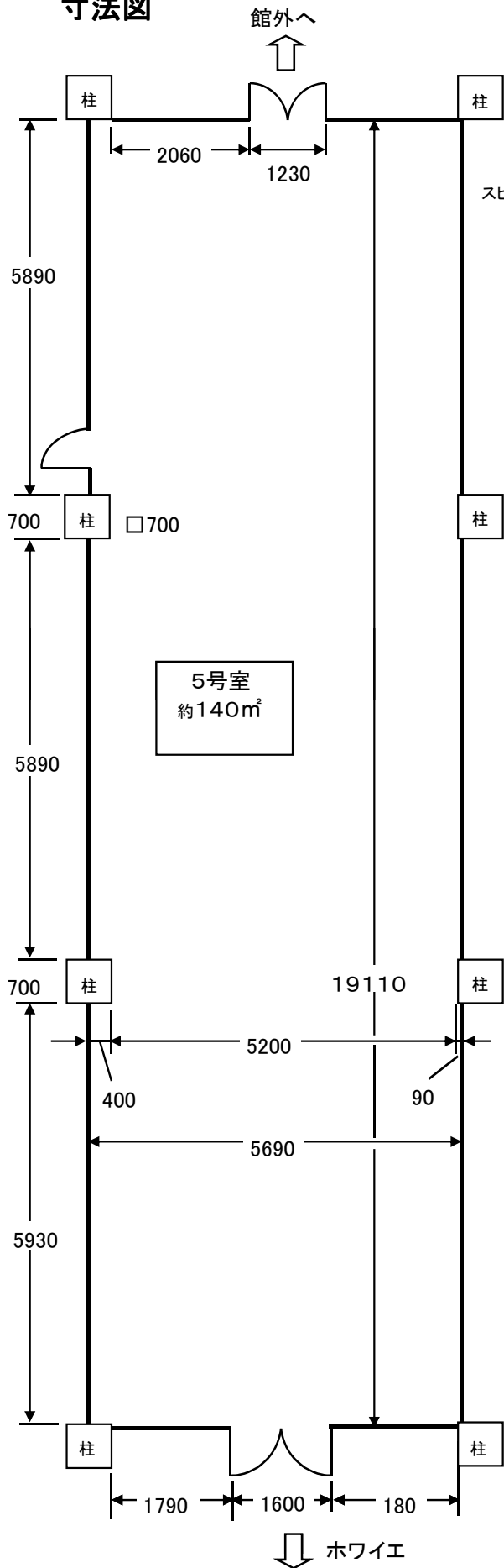
寸法図
